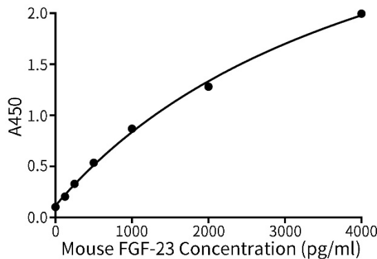
图3. Mouse FGF-23 ELISA Kit的标准曲线。实测数据会因实验条件、检测仪器等的不同而存在差异，图中数据仅供参考。
